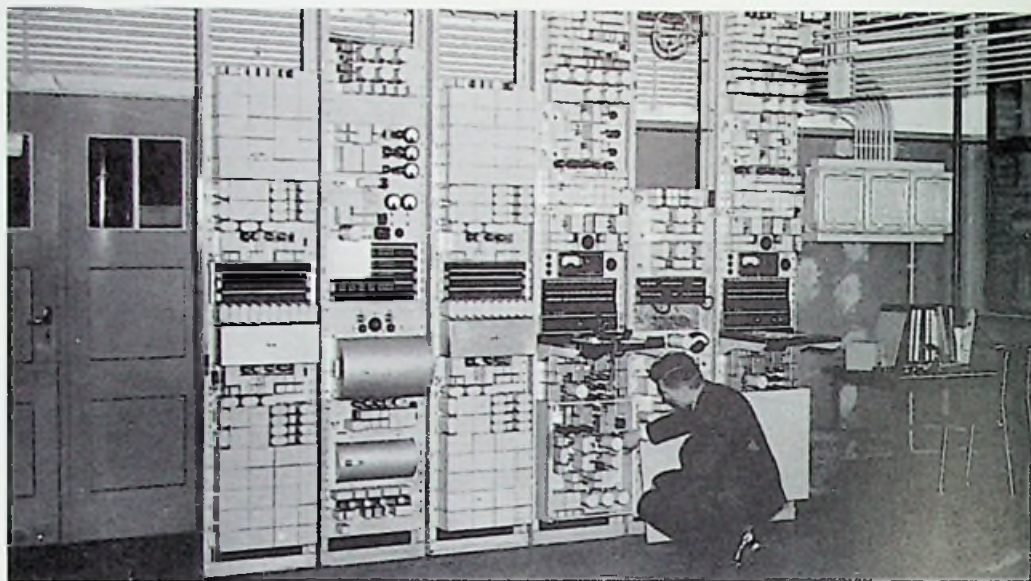
Radiovorken met scramblingsysteem voor geheimtelefonie met Noord-Amerika
