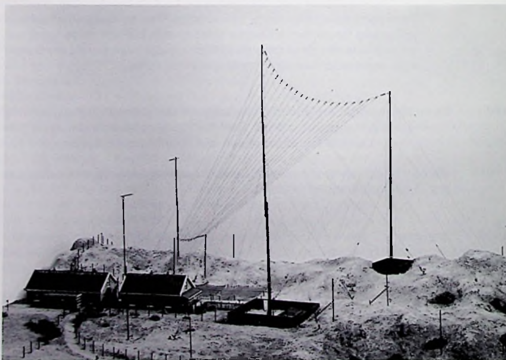
Kuststation Scheveningen-Haven met harp-antenne 1904-1910
